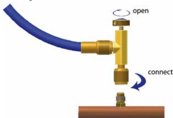
Schema di Connessione Connecting scheme
